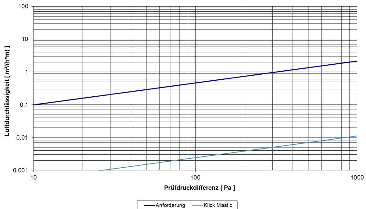
Abbildung 4: Luftdurchlässigkeit (WDI ISO FIRE 100 Mastic)
