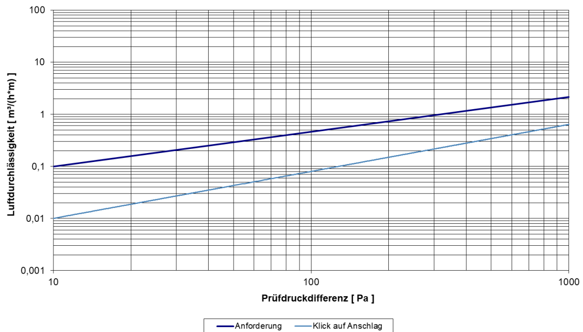
Abbildung 4: Luftdurchlässigkeit (WDI ISO COOL 100)
