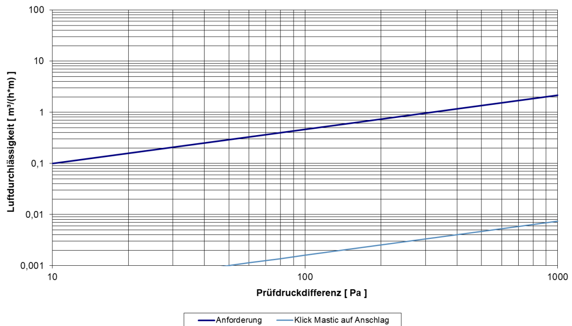
Abbildung 4: Luftdurchlässigkeit (WDI ISO COOL 100 Mastic)
